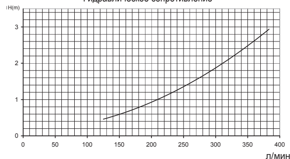
Гидравлическое сопротивление
